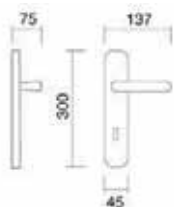
Art. 3740 Maniglia su placca Handle on plate
