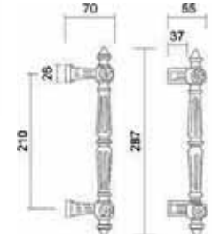
Art. 0550 Maniglione Pull handle
