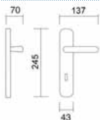
Art. 3480 Maniglia su placca Handle on plate
