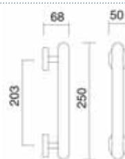
Art. 3075 Maniglione Pull handle
