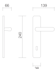
Art. 1020 Maniglia su placca Handle on plate
