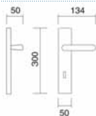
Art. 3670/3540 Maniglia su placca Handle on plate
