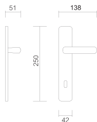
Art. 3760/ Maniglia su placca Handle on plate
