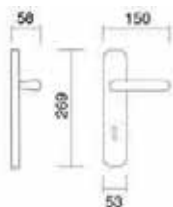
Art. 3360 Maniglia su placca Handle on plate
