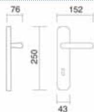
Art. 3290 Maniglia su placca Handle on plate
