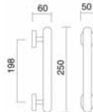
Art. 3085 Maniglione Pull handle
