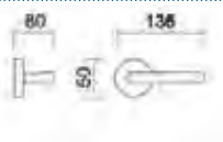
Art. 2781 Maniglia su rosetta Handle on rose
