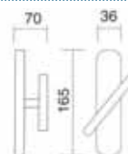
Art. 2868 Dreh kipp Dreh kipp
