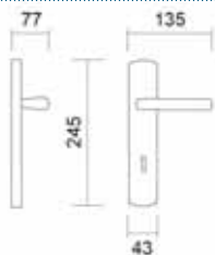
Art. 3250 Maniglia su placca Handle on plate
