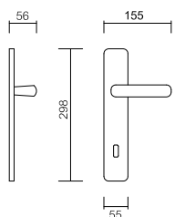
Art. 3810 Maniglia su placca Handle on plate
