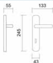
Art. 3380 Maniglia su placca Handle on plate
