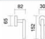
Art. 3058 Dreh kipp Dreh kipp
