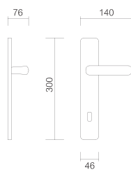
Art. 2016/3740 Maniglia su placca Handle on plate
