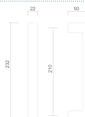
Art. 3875 Maniglione Pull Handle
