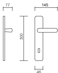
Art. 3820 Maniglia su placca Handle on plate
