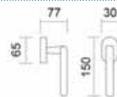
Art. 3258 Dreh kipp Dreh kipp
