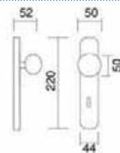
Art. 1446 Pomolo su placca Knob on plate
