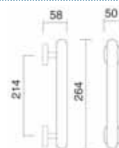
Art. 2865 Maniglione Pull handle
