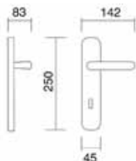
Art. 2840 Maniglia su placca Handle on plate
