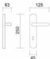
Art. 1010 Maniglia su placca Handle on plate
