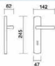
Art. 3230 Maniglia su placca Handle on plate
