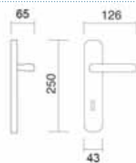
Art. 2950 Maniglia su placca Handle on plate
