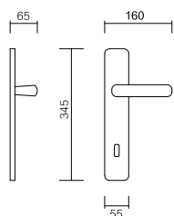
Art. 3920 Maniglia su placca Handle on plate
