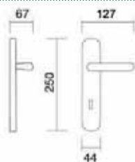
Art. 1440 Maniglia su placca Handle on plate
