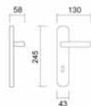
Art. 3470 Maniglia su placca Handle on plate
