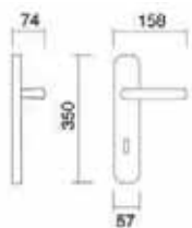
Art. 3780 Maniglia su placca Handle on plate
